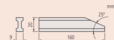
Plain jaw : 619018
