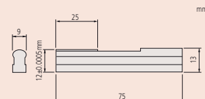
Half-round jaw : 619013
