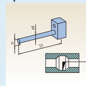
Small hole : 12AAE299 Tip shape : Single bevel Tip angle : 20° Tip radius : 25 µm Tip material : Carbide
