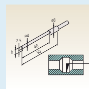
Small hole : 932695 / 12AAE875 Tip shape : Single bevel / Cone Tip angle : 20° / 30° Tip radius : 25 µm / 25 µm Tip material : Carbide / Carbide
