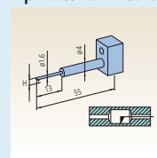
Small hole : 12AAE297 Tip shape : Single bevel Tip angle : 20° Tip radius : 25 µm Tip material : Carbide
