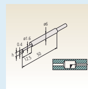
Small hole : 932693 / 12AAE873 Tip shape : Single bevel / Cone Tip angle : 20° / 30° Tip radius : 25 µm / 25 µm Tip material : Carbide / Carbide
