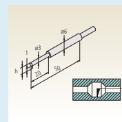
Small hole : 932694 / 12AAE874 Tip shape : Single bevel / Cone Tip angle : 20° / 30° Tip radius : 25 µm / 25 µm Tip material : Carbide / Carbide
