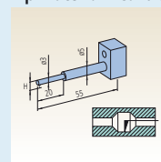
Small hole : 12AAE298 Tip shape : Single bevel Tip angle : 20° Tip radius : 25 µm Tip material : Carbide
