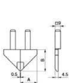
Стандартные губки
