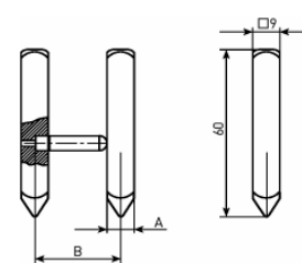
Разметочные губки
