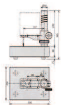
957460 Компаратор (стенд)
