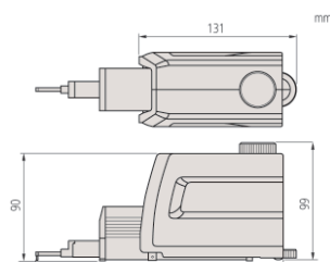
SJ-411: 207,5 мм / SJ-412: 234 мм Приводной блок
