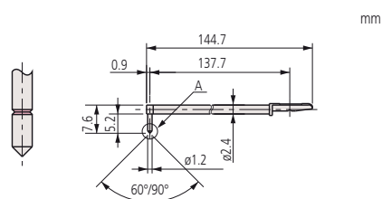
Щуп для глубоких отверстий [тройной длины]
