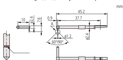
Щуп для дна глухого отверстия
