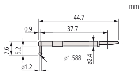
Щуп для глубоких канавок 40 мм
