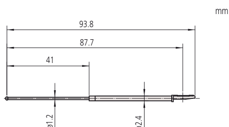
Щуп для контроля шероховатости и волнистости цилиндрических деталей (требуется 178-611)
