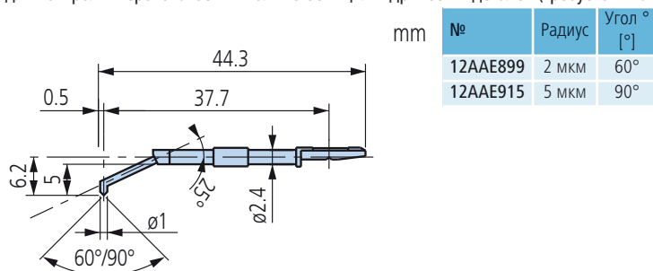
Щуп для контроля шероховатости и волнистости цилиндрических деталей (требуется 178-611)
