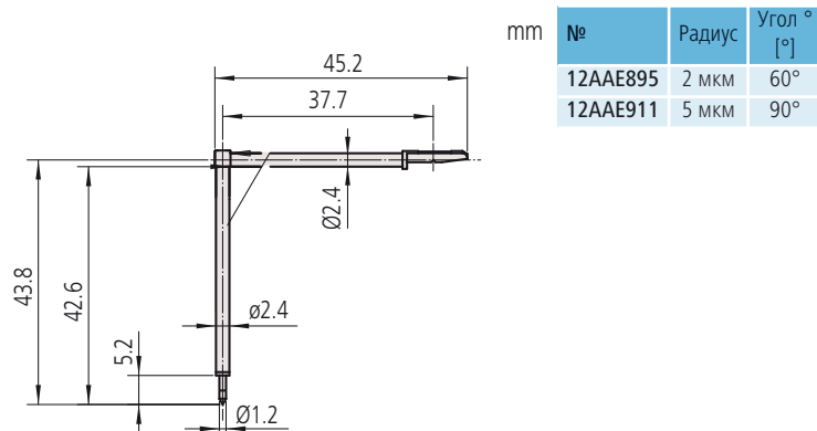
Щуп для глубоких канавок 40 мм
