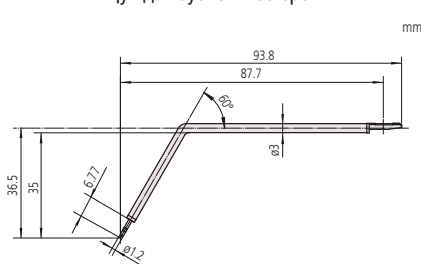
Щуп для зубьев шестерен [двойной длины]
