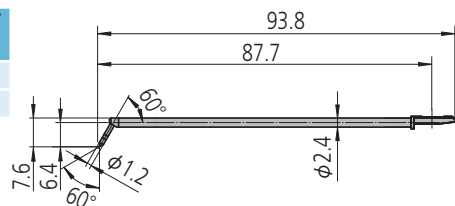
Щуп для угловых отверстий [двойной длины]
