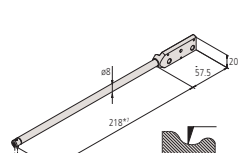
Прямая консоль CV-3200/CV-4500 SV-C3200/SV-C4500 SV-C4500CNC
