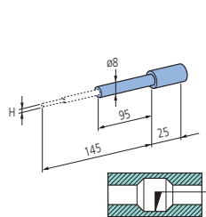
Консоль с щупом для малых отверстий CV-2100
