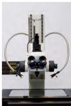
Двойной S-образный световод
