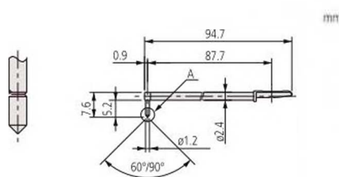
Для глубоких отверстий [двойной длины]
