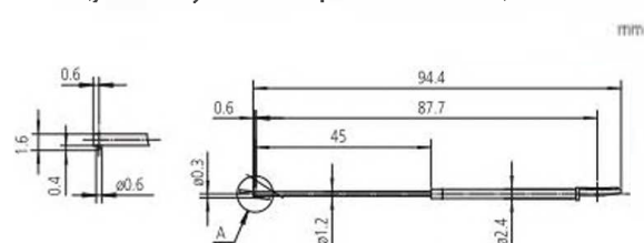
Щуп для глубоких отверстий [двойной длины]
