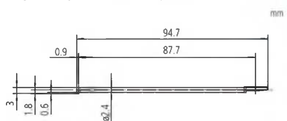
Щуп для глубоких малых отверстий [двойной длины]
