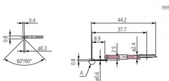
Для сверхмалых отверстий
