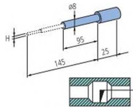
Консоль с щупом для малых отверстий CV-2100
