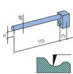
Прямая консоль CV-2100
