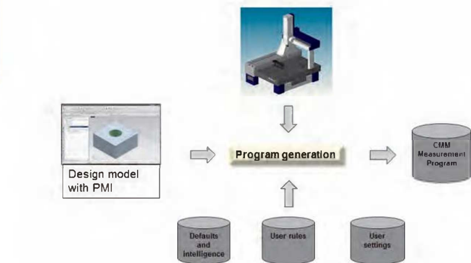
Последовательность выполняемых действий в MiCAT Planner
