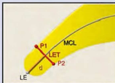
Передняя кромка - толщина на заданном расстоянии
