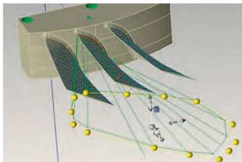
Оптимизация траектория перемещения щупа
