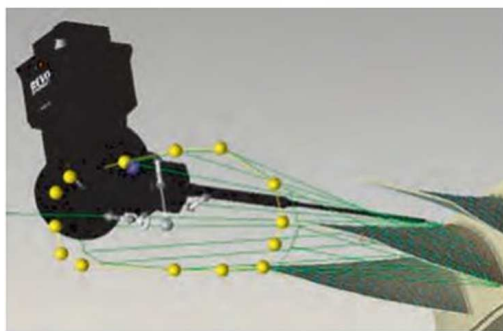
Установка сечений на CAD-модели
